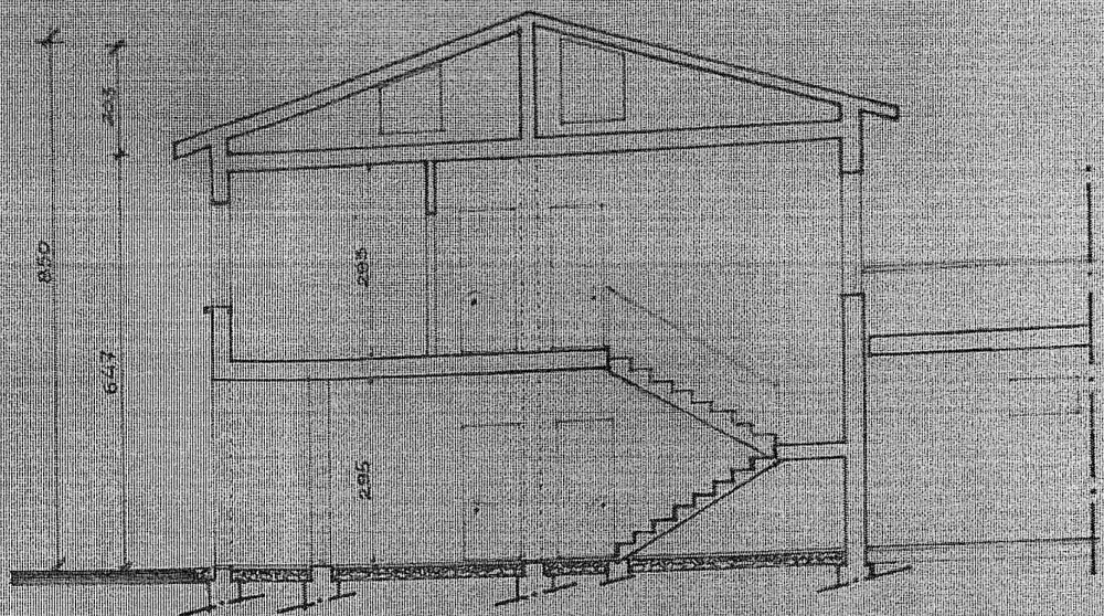
sezione B-C
